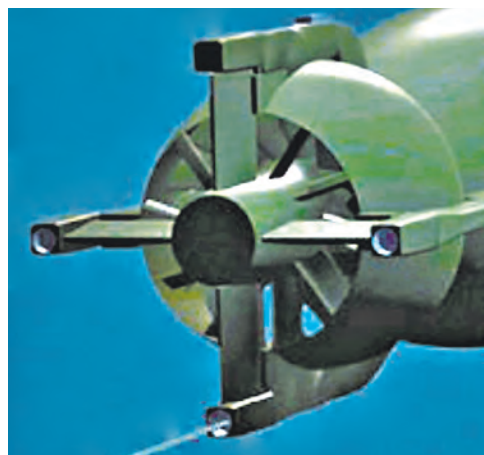
Выход кабеля телеуправления
