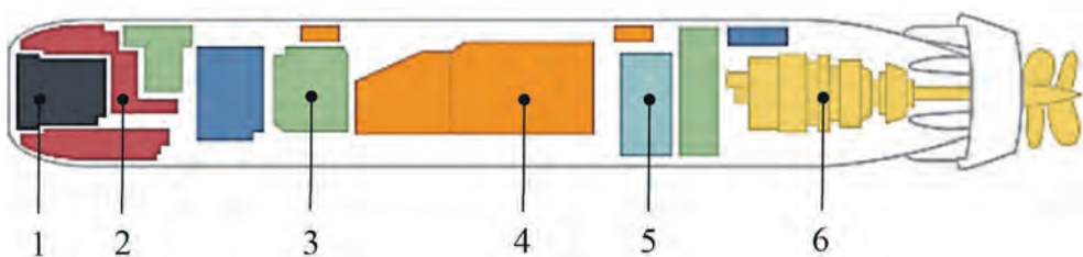
Модульные элементы торпеды TR45: 1 – ГСН; 2 – ССН; 3 – система управления подрывом БЧ; 4 – аккумуляторная батарея; 5 – система управления двигателем; 6 – электродвигатель
