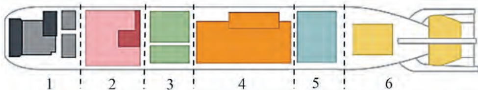
Модули торпеды TS47: 1 – модуль ГСН и модуль обработки ГА-сигналов и формирования ДНА; 2 – модуль боевого зарядного отделения с системой управления подрывом БЧ или практическим модулем; 3 – модуль ССН; 4 – аккумуляторная батарея; 5 – модуль системы телеуправления и катушка с кабелем; 6 – электродвигатель с движителем «Памп-Джет»
