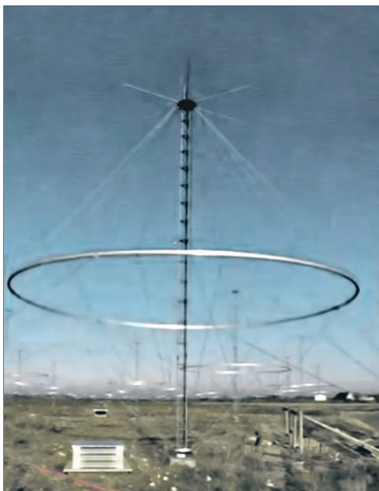
Биконический элемент загоризонтной радиолокационной станции «Нострадамус»
