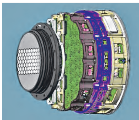
Активно-пассивная ГСН MS4
