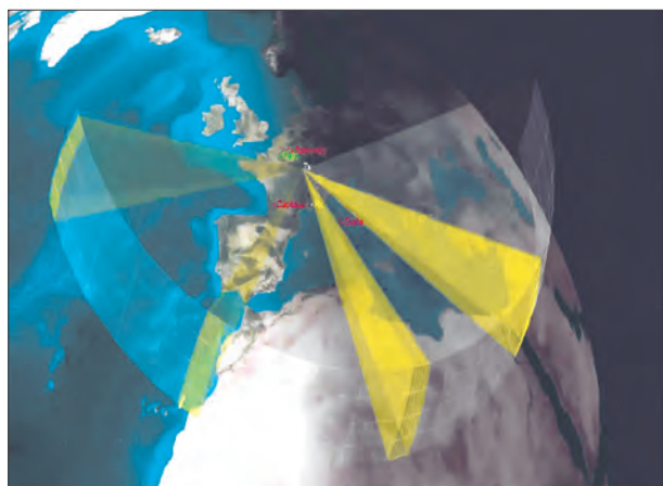
Общий вид зоны космического пространства, контролируемой РЛС «Грав»
