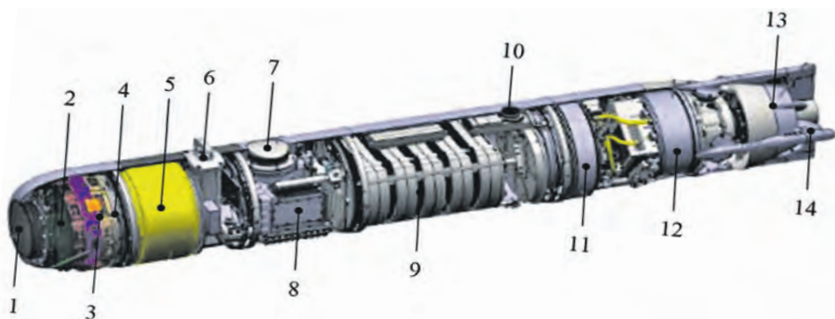
Активно-пассивная ГСН MS4
