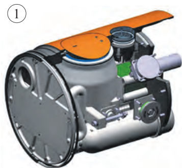
Практический модуль торпеды TS47: 1 – вид в разрезе; 2 – воздушный поплавок, обеспечивающий всплытие
